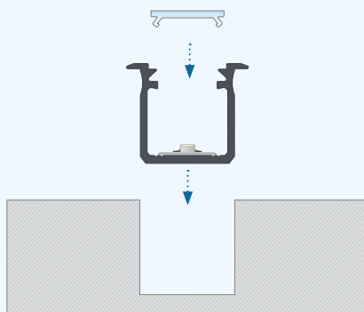
PL Instrukcja montażu profilu G wpuszczanego z kloszem BASIC.
