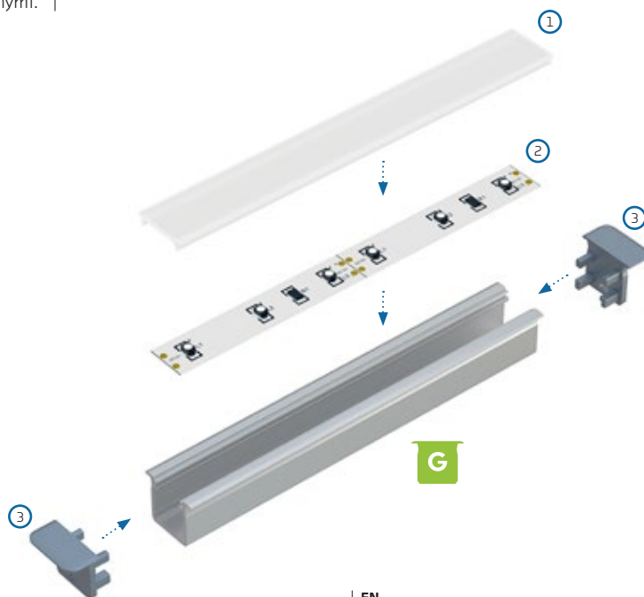
PL Schemat złożenia elementów systemu oświetleniowego z wykorzystaniem profilu G oraz [1] klosza BASIC, [2] taśmy LED, [3] zaślepek z otworami.
