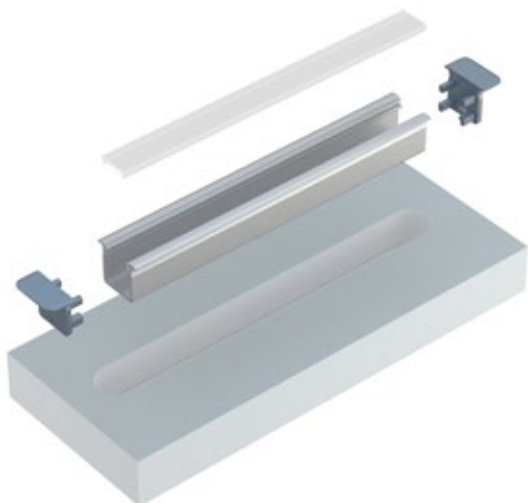
PL Rzut aksonometryczny przed montażem profilu G wewnątrz wyfrezowanego otworu z kloszem BASIC oraz zaślepkami bocznymi.
